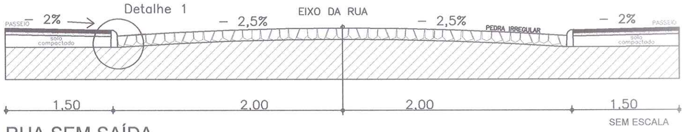
RUA SEM SAÍDA CORTE B B' SEM ESC.
